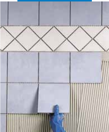
Egyszer égetett burkolólap ragasztása gipszkartonra
