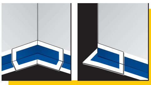
90°-os sarok elhelyezése 270°-os sarok elhelyezése
